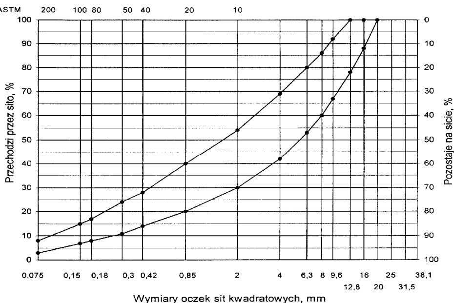
Rys. 2. Krzywe graniczne uziarnienia mieszanki mineralnej BA od 0 do 16 mm dla warstwy wiążącej, wyrównawczej i wzmacniającej nawierzchni drogi o obciążeniu ruchem KR1 lub KR2
